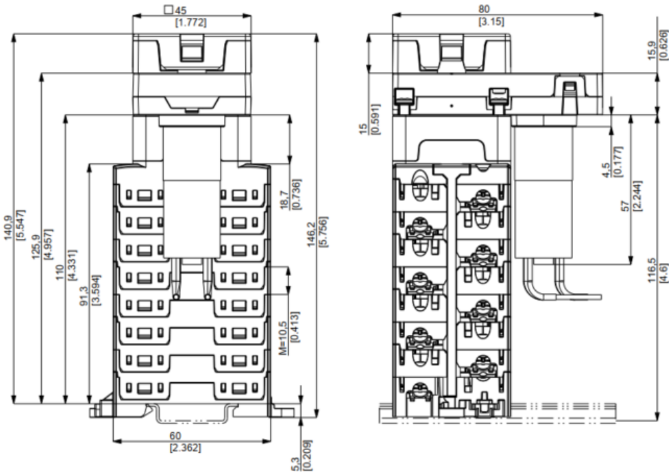
Dimensions
